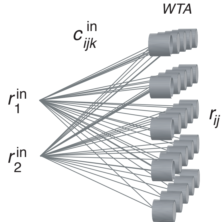
A. 2-d feature space and SOM layer
