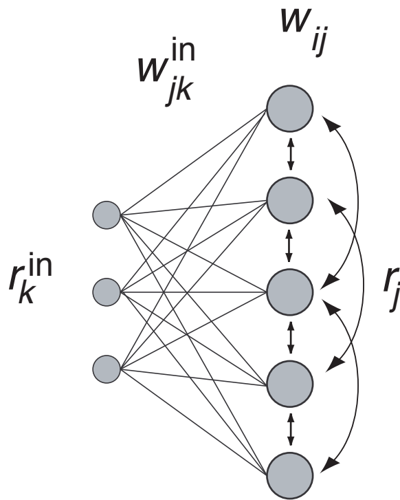
B. 1D feature space and SOM layer
